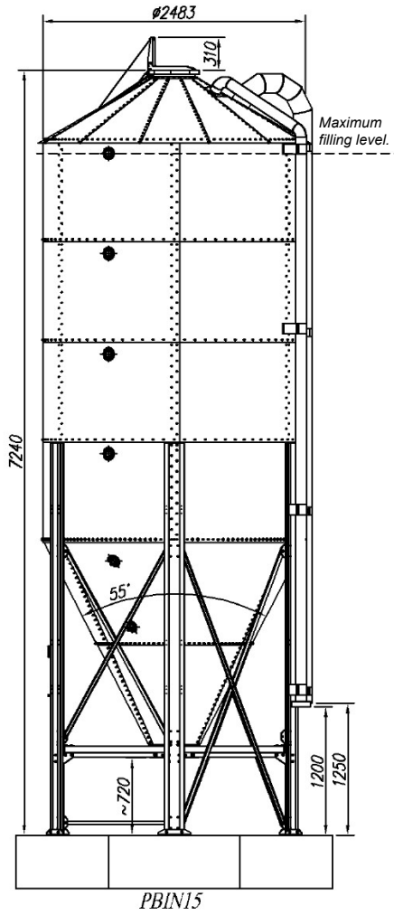
Lopbarības torņu PBIN izmēri
