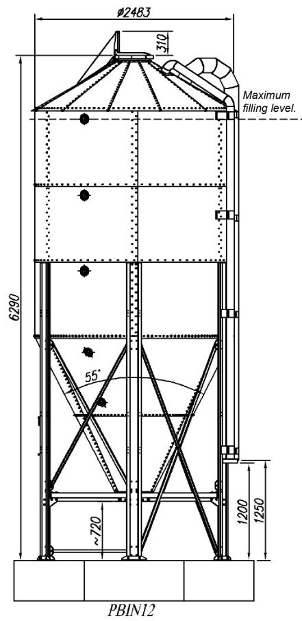
Lopbarības torņu PBIN izmēri
